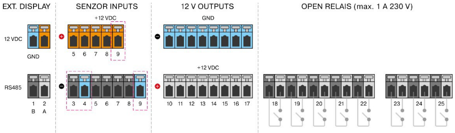
Fig. 2. Terminalboksen
